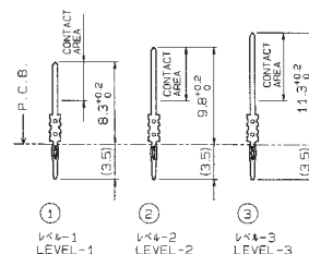
コンタクト寸法 CONTACT DETAIL
