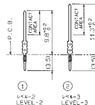
コンタクト寸法 CONTACT DETAIL
