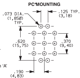
7301MD9__BE 3PDT
