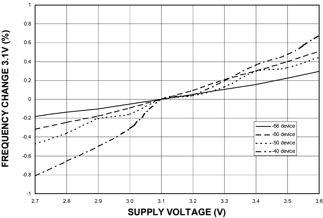
DS1077L VOLTCO
