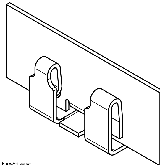
シールドロック嵌合状態斜視図 SHIELD LOCK MATING
