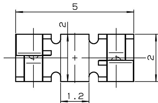
推奨パターンレイアウト RECOMMENDED PATTERN LAYOUT
