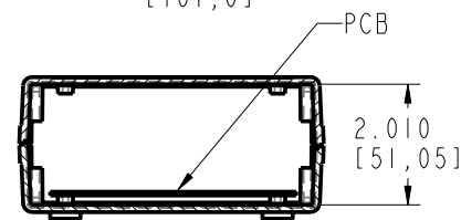
SECTION B-B CM5-200
