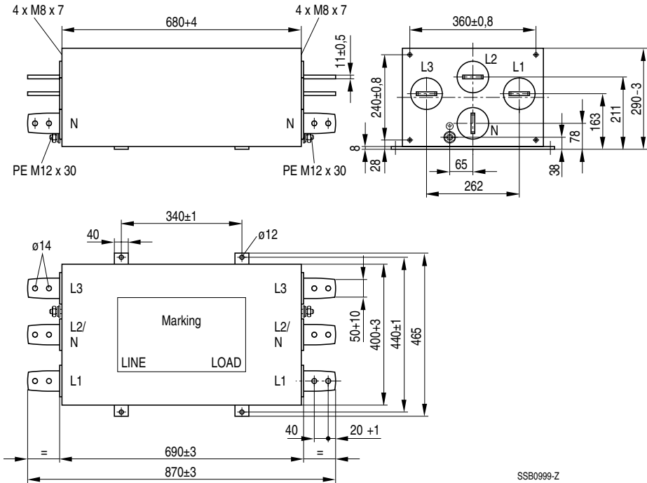
Maßbild B84144-G1600-S
