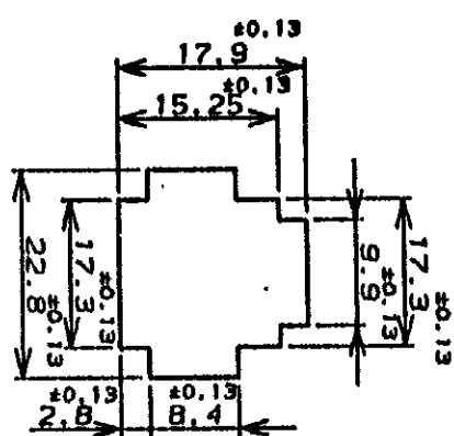
パネル取付穴寸法 FIG. 1
