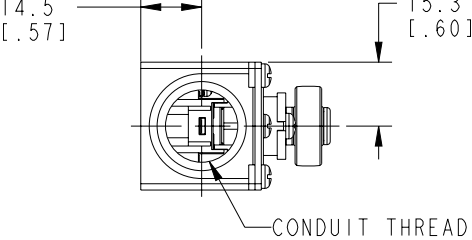
Figure 22. GLD Conduit
