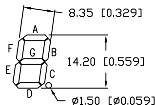
DIGIT DETAIL
