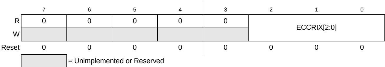
Figure 8-8. FECCR Index Register (FECCRIX)
