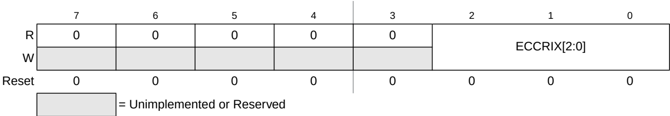
Figure 10-8. FECCR Index Register (FECCRIX)
