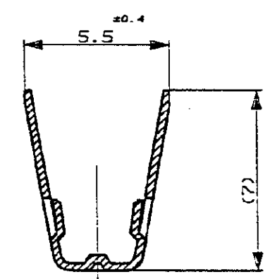
SECT. 断面 C-C
