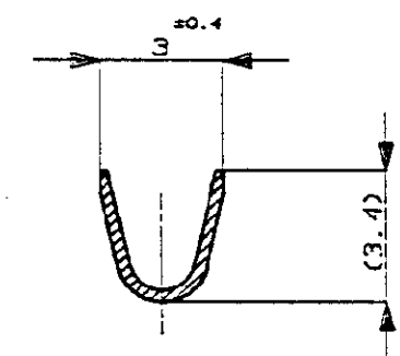
SECT. 断面 B-B
