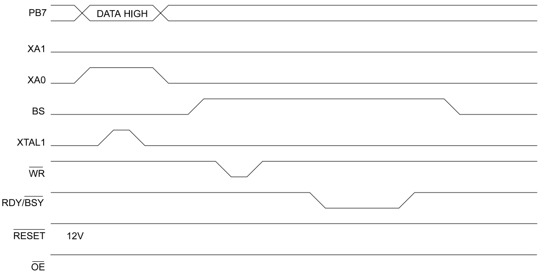
图 32 编程波形二
