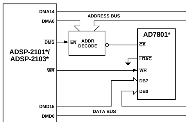
Figure 29. AD7801-ADSP-2101/ADSP-2103 Interface
