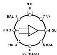
TO-99 (J-Suffix)
