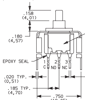
8121SD3_GE SPDT
