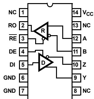
ISL32452E, ISL32455E
