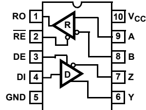
ISL32450E, ISL32453E
