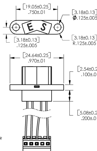
OPB755TZ
