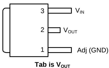
(3) TO220-3L
