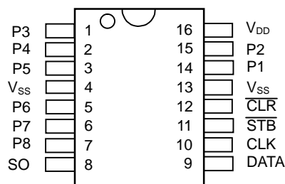
NJU3712D/M
