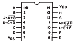
CD4001B
