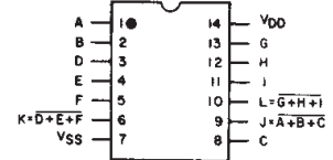
CD4025B
