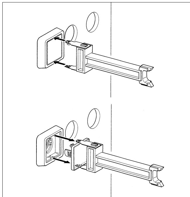
Lampenwechsel von vorne
