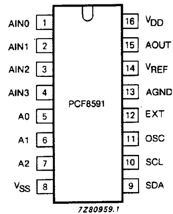
Fig.2 Pinning diagram.
