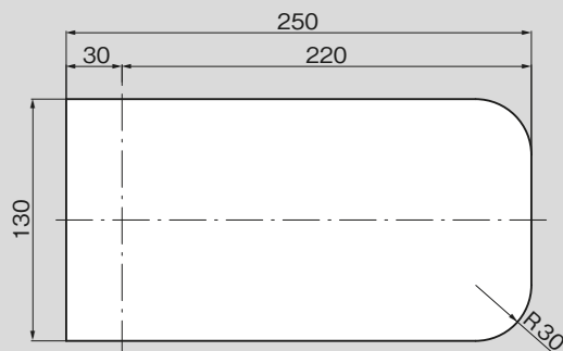
パネル穴明け寸法 Panel drilling dimensions
