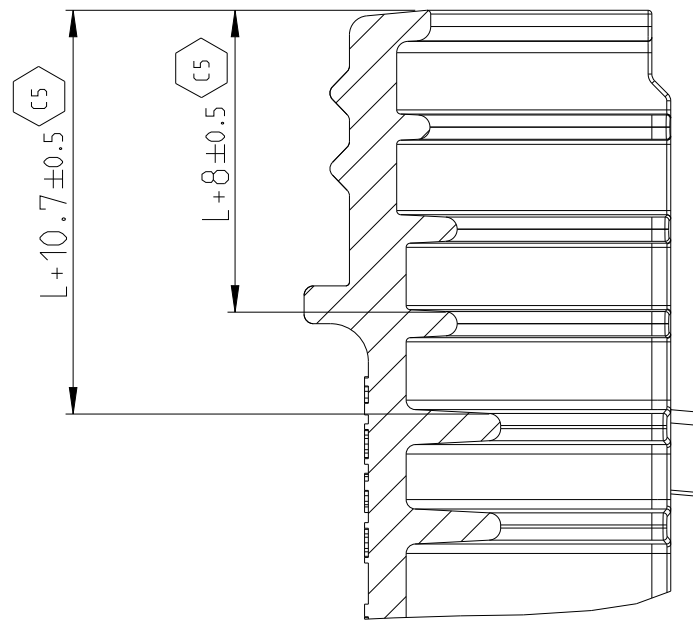
L+ = ADD LENGTH FOR CORRUGATED TUBE zus. Länge des Wellrohrs
