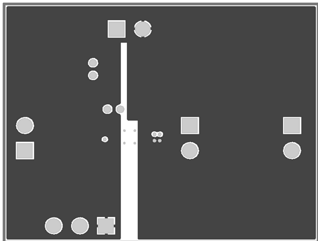
Internal Layer 2
