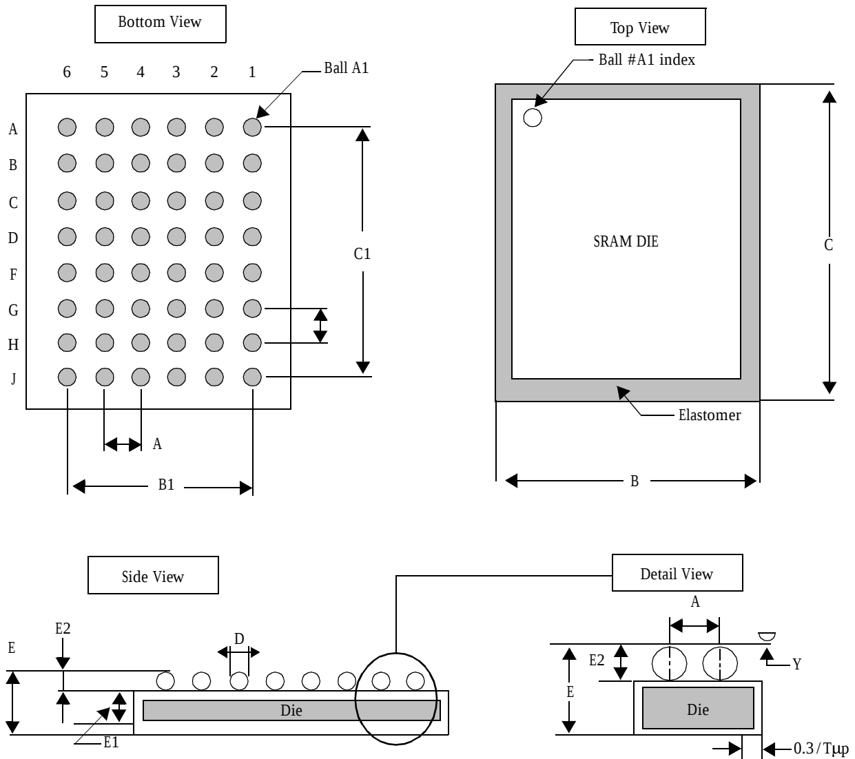
48-ball FBGA
