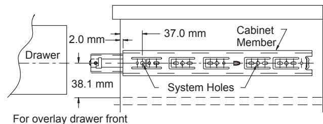
Figure 2 32 mm System—Cabinet
