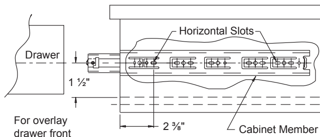
Figure 2 32 mm System—Cabinet
