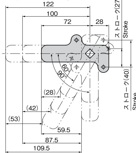
作動図 Operation drawings
