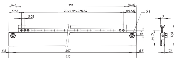
2) Press-in insert M4
