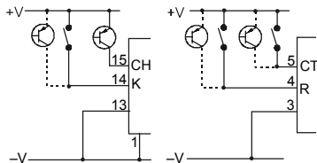
Entrées (PNP)
