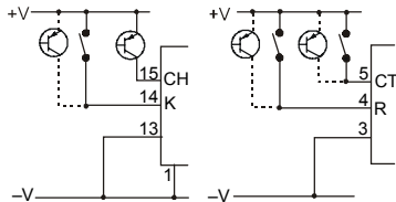
Entrada tipo Source (PNP)
