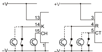
Entrées (NPN)
