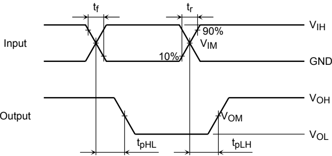
図 2 t_{pLH} , t_{pHL}
