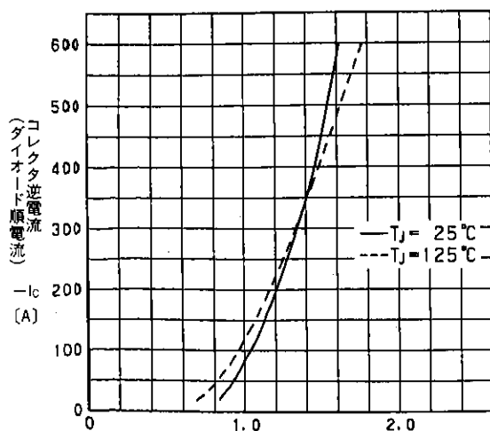
エミッタ・コレクタ間電圧 V_{ECO} (V) (ダイオード順電圧) 高速フリーホイーリングダイオード順電圧特性 Forward Voltage of Free Wheeling Diode
