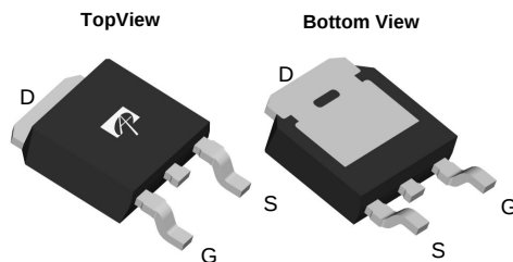
TO252 DPAK
