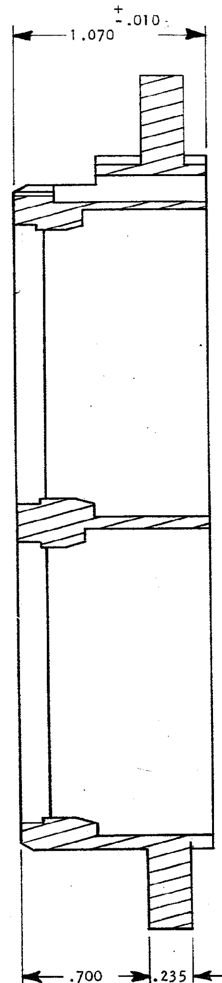
SECTION A-A
