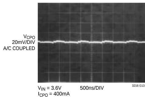
2x Mode CPO Output Ripple
