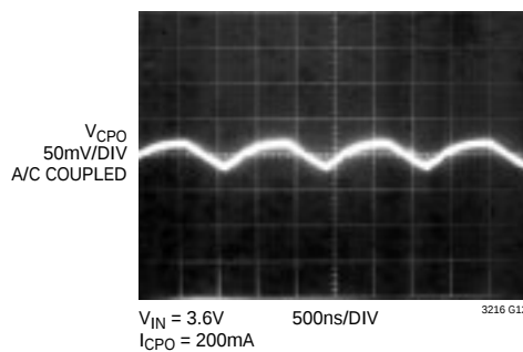
1.5x Mode CPO Output Ripple
