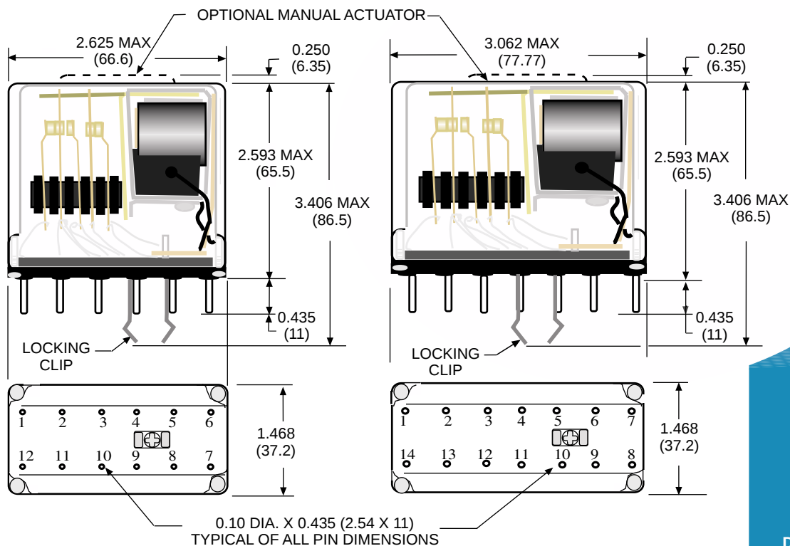
219XBX DPDT
