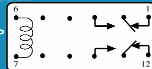
219XBX DPDT
