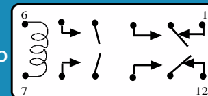
219BBXP DPDT+2 NO
