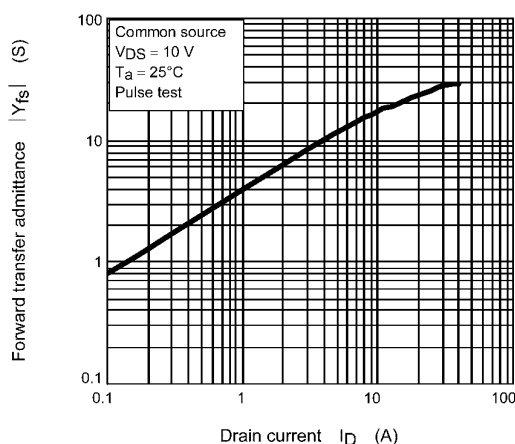
Fig. 8.5 |Y_{fs}| - I_D
