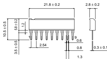
SIP9
