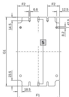
Montageplatte
