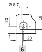
Ansicht A für Wandbefestigung
