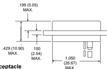
Receptacle
