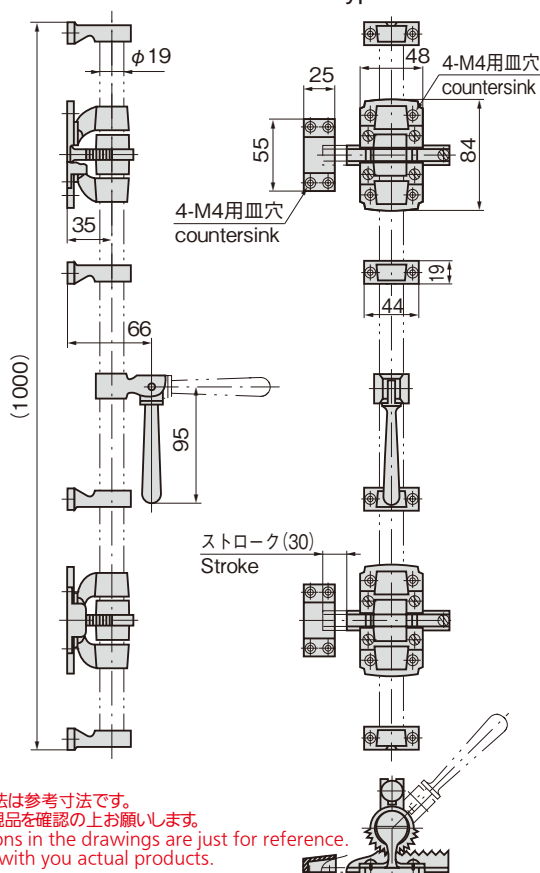
〔FA-807-2 両開き用・オフセットタイプ〕 Both-side use・Offset type
