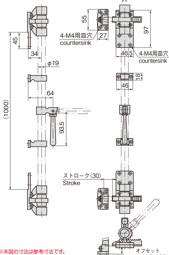
〔FA-807-2 両開き用・オフセットタイプ〕 Both-side use・Offset type
