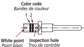
Male Contact / Contact mâle
