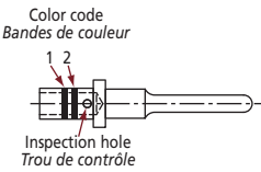
Male Contact / Contact mâle
