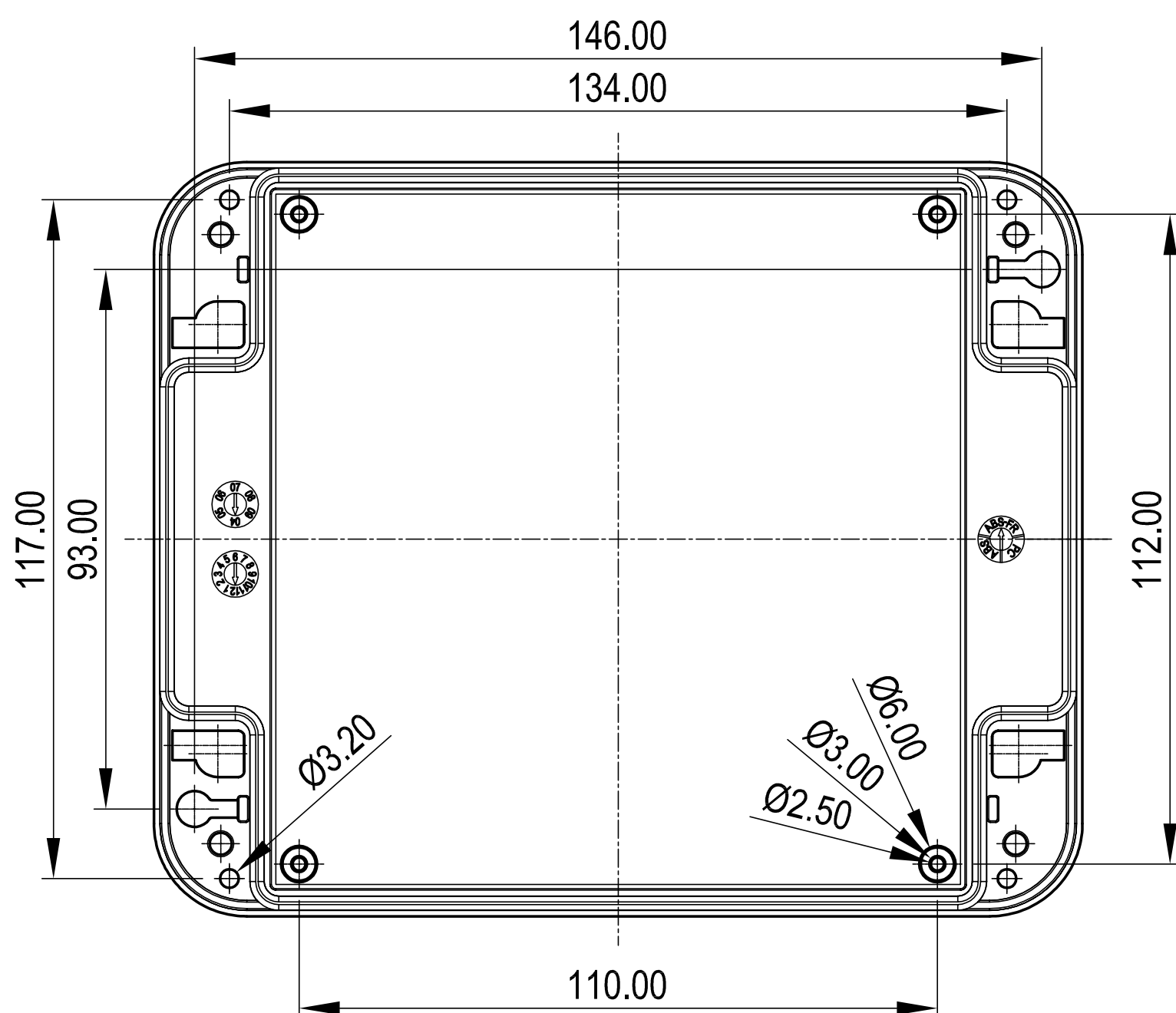
Oberteil Innenansicht Top part inside view
