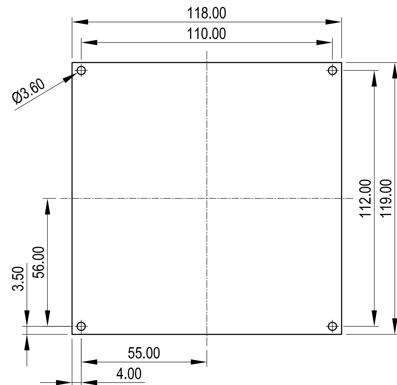
Platine Oberteil PCB top part
