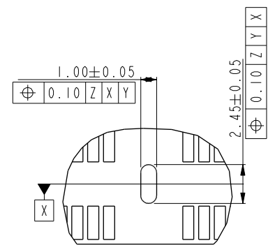
Center forklock type
