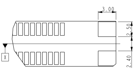
DETAIL E SCALE 3.000
