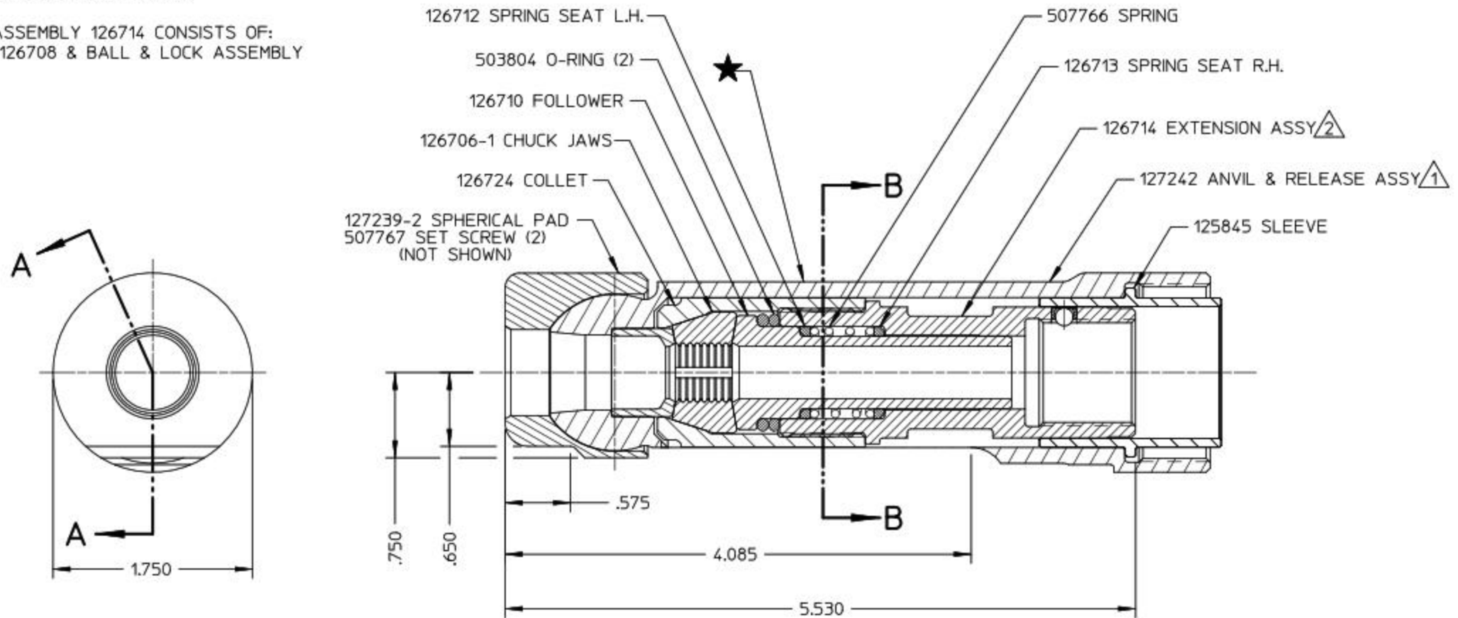
SECTION A-A
