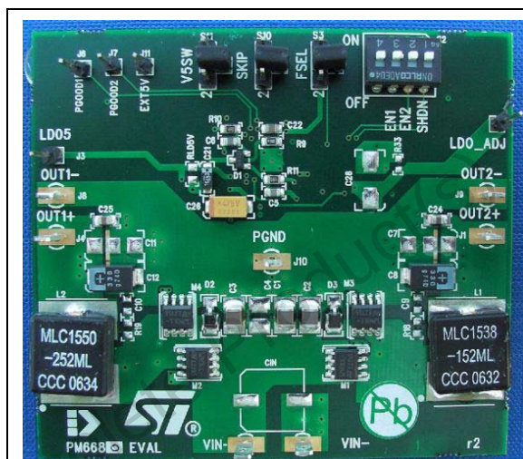
STEVAL-ISA053V1
