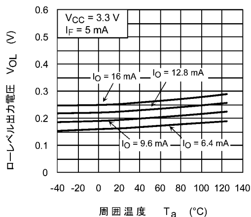
図 12.2.4 V_{OL} - T_a
