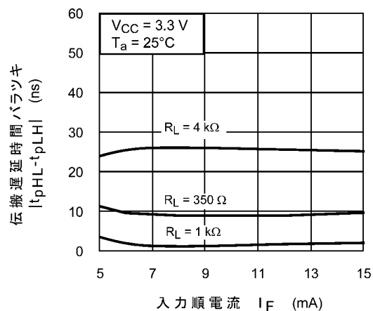
図 12.2.18 |t_{pHL} - t_{pLH}| - I_F
