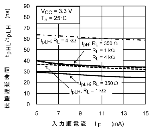
図 12.2.17 t_{pHL}, t_{pLH} - I_F
