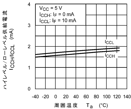
図 12.2.9 I_{CCH}, I_{CCL} - T_a
