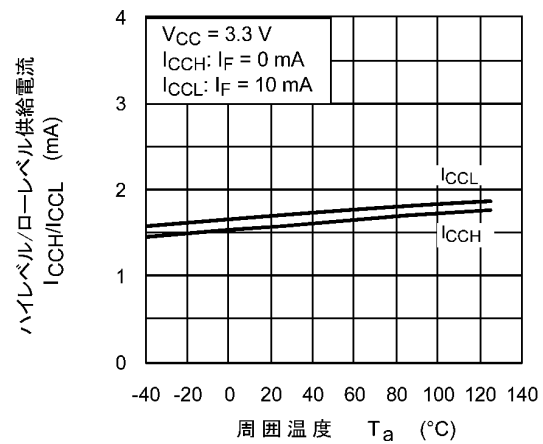
図 12.2.10 I_{CCH}, I_{CCL} - T_a
