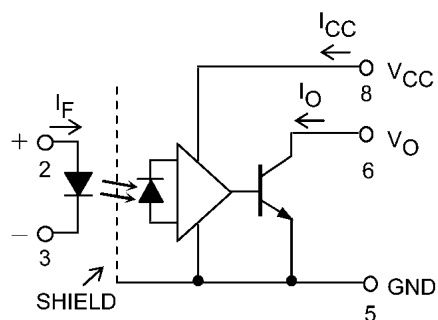
図 5.1 内部回路構成
