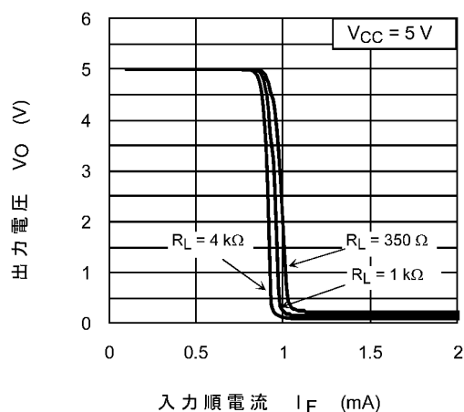
図 12.2.5 V_O - I_F
