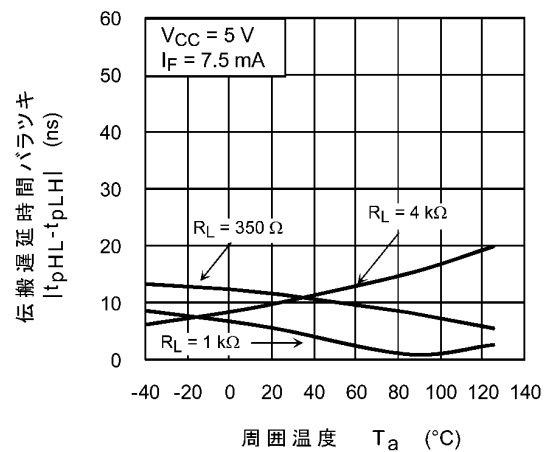
図 12.2.12 |t_{pHL} - t_{pLH}| - T_a
