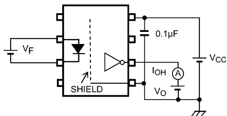
図 12.1.1 I_{OH} 測定回路
