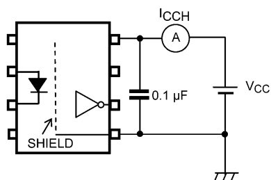
図 12.1.3 I_{CCH} 測定回路
