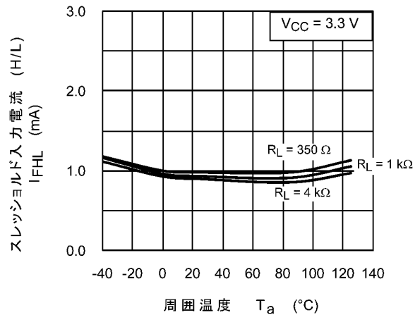
図 12.2.8 I_{FHL} - T_a
