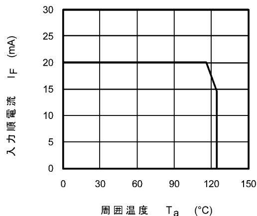
図 12.2.2 I_F - T_a
