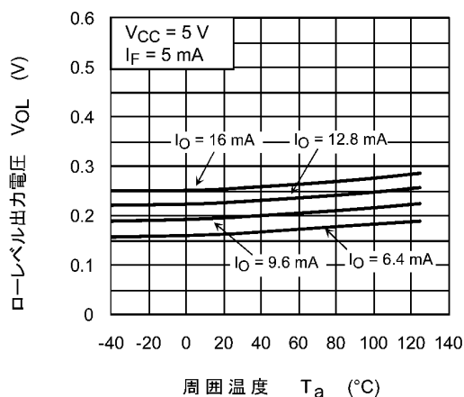
図 12.2.3 V_{OL} - T_a
