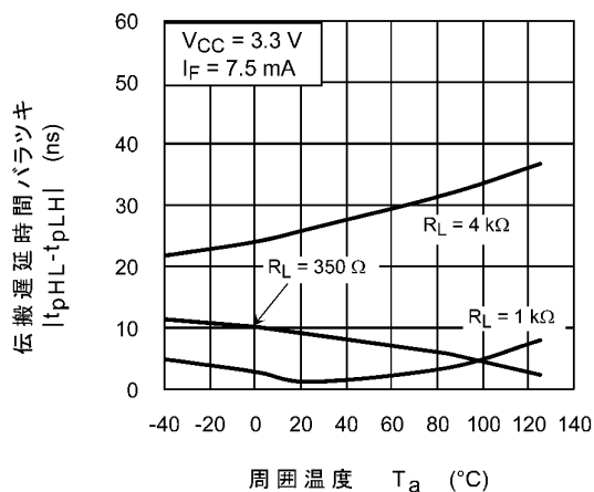
図 12.2.14 |t_{pHL} - t_{pLH}| - T_a
