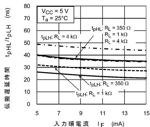
図 12.2.15 t_{pHL}, t_{pLH} - I_F
