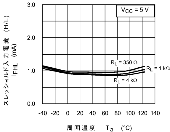
図 12.2.7 I_{FHL} - T_a
