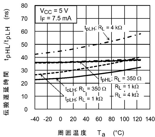
図 12.2.11 t_{pHL}, t_{pLH} - T_a
