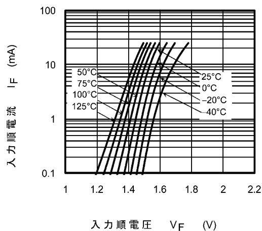
図 12.2.1 I_F - V_F
