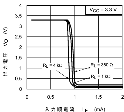
図 12.2.6 V_O - I_F
