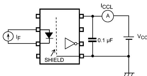
図 12.1.4 I_{CCL} 測定回路
