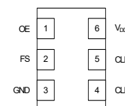
Si513 LVDS/LVPECL/HCSL/CMOS Dual XO
