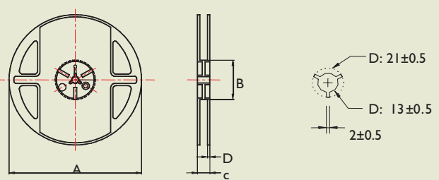
Reel Dimensions
