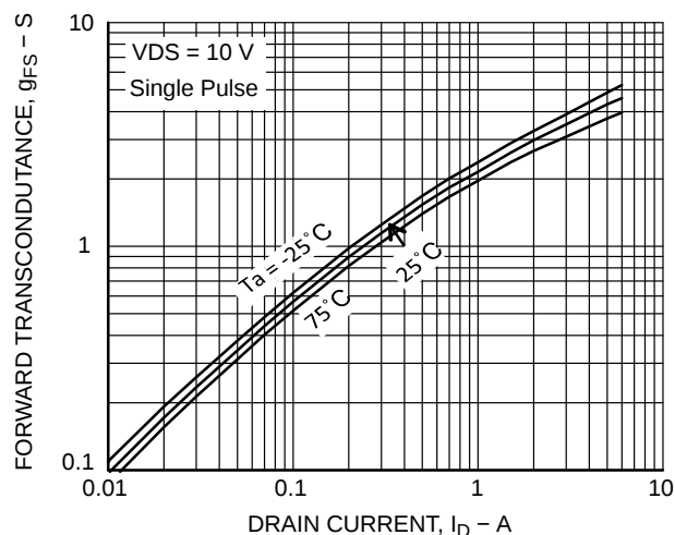
Figure 6. g_{FS} - I_D
