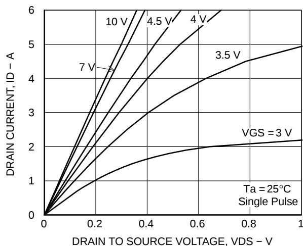
Figure 2. I_D - V_{DS}
